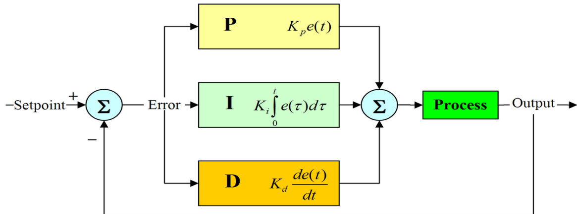
PID 控制器的方塊圖
